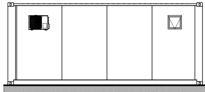
ELEVACION POSTERIOR
