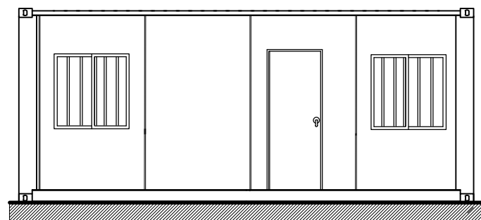
ELEVACION PRINCIPAL
