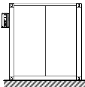
ELEVACION LATERAL IZQUIERDA
