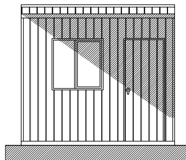
ELEVACION PRINCIPAL
