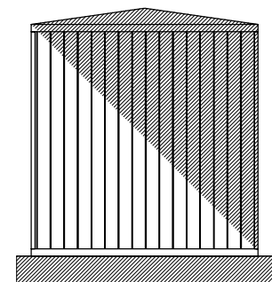
ELEVACION LATERAL DERECHA
