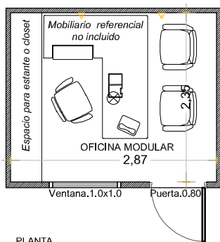
PLANTA
