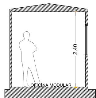
CORTE TRANSVERSAL
