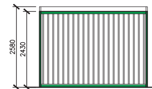
ELEVACIÓN NORTE
