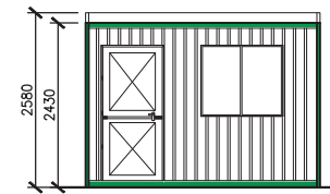
ELEVACIÓN SUR
