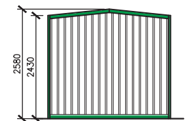
ELEVACIÓN OESTE
